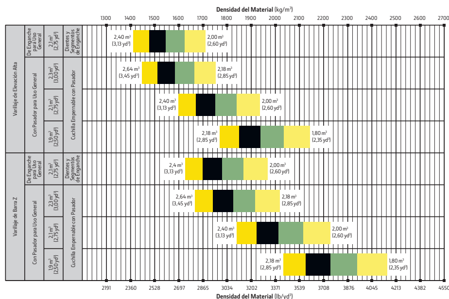
Factores de Llenado del Cucharón
